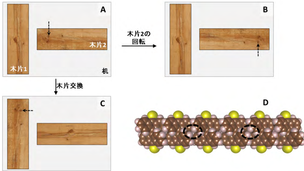
図 4. (A–C) 机の上に置いた木片で回転・交換の対称性を説明する。点線の矢印は対称性を下げる欠点を示す。(D) 数理フレームワークで予想された鎖構造。黒い円(点線)は欠陥を示す。欠陥の導入により対称性が下がり、鎖構造のエントロピーが上がることによって、鎖構造が形成される。
